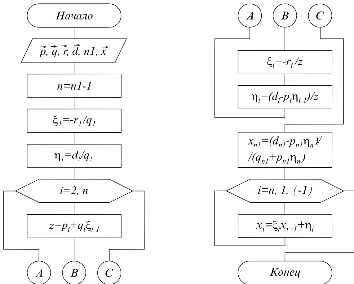
Рис. 15.2 Схема алгоритма метода прогонки
