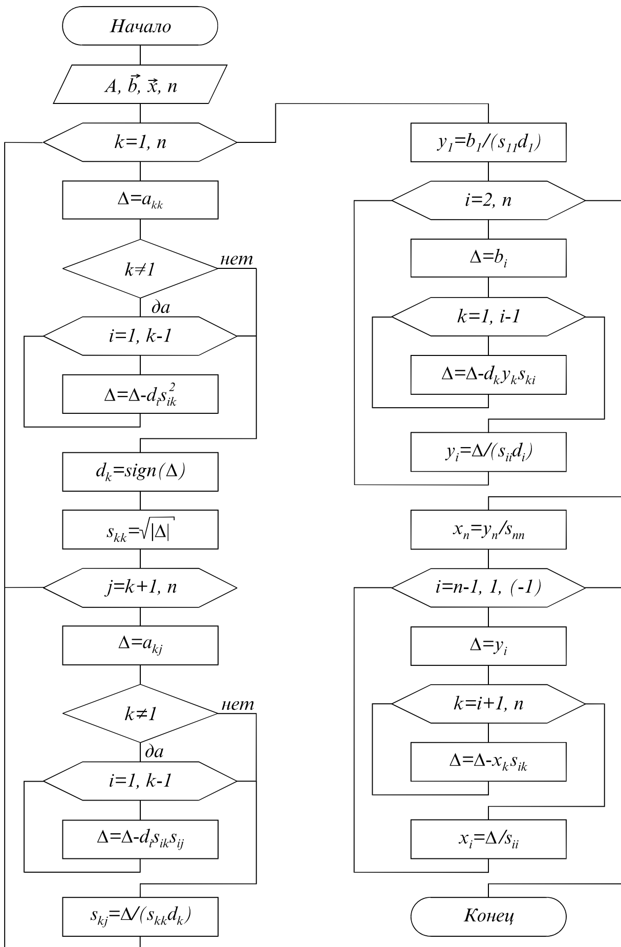
Рис. 15.3 Схема алгоритма метода квадратного корня
