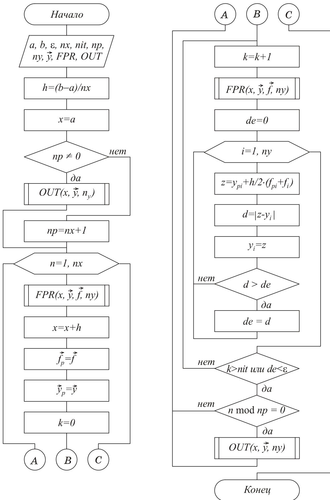
Рис. 19.3 Схема Рунге-Кутты 2-го порядка
