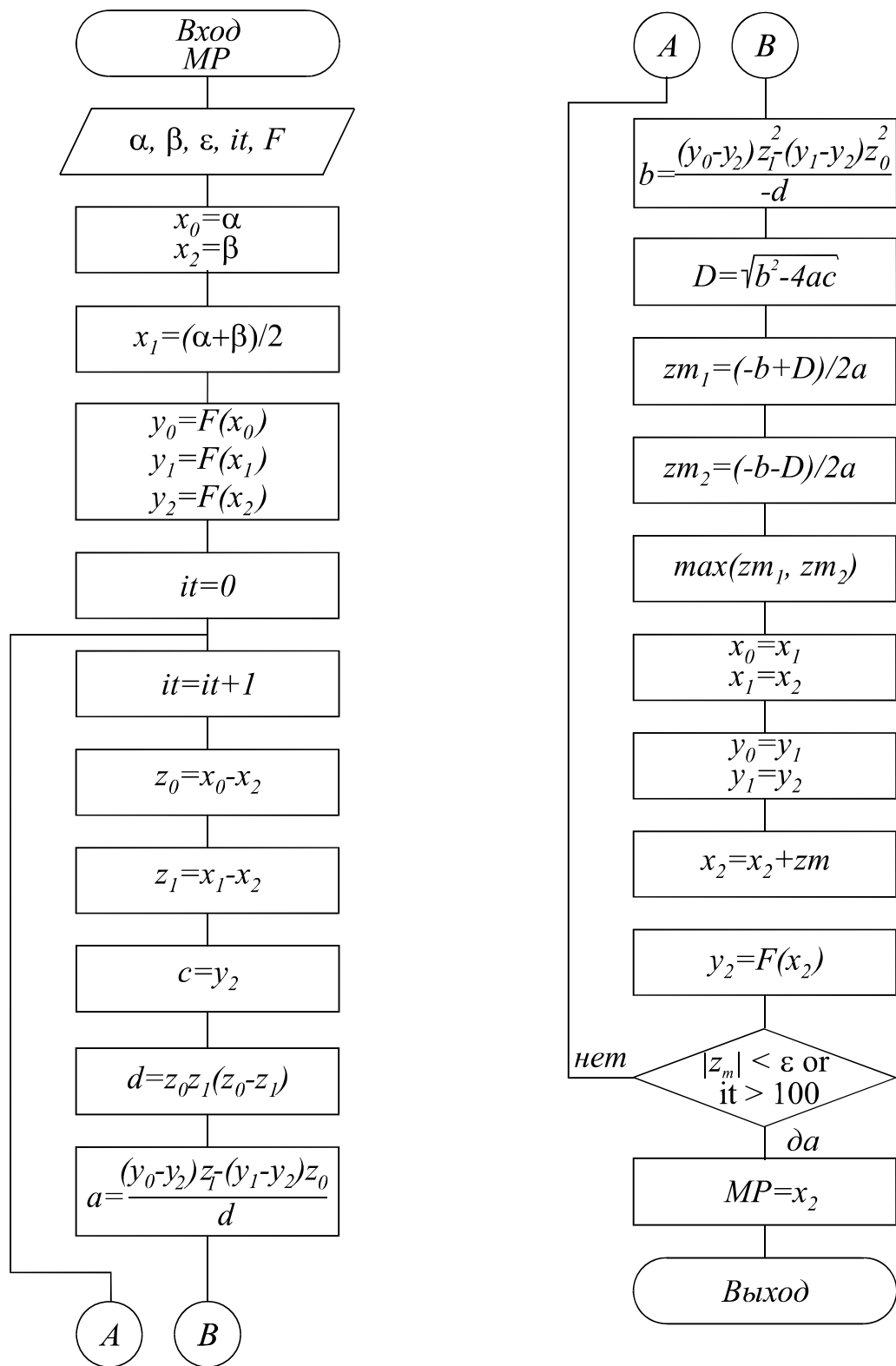
Рис. 17.3 Схема алгоритма метода парабол
