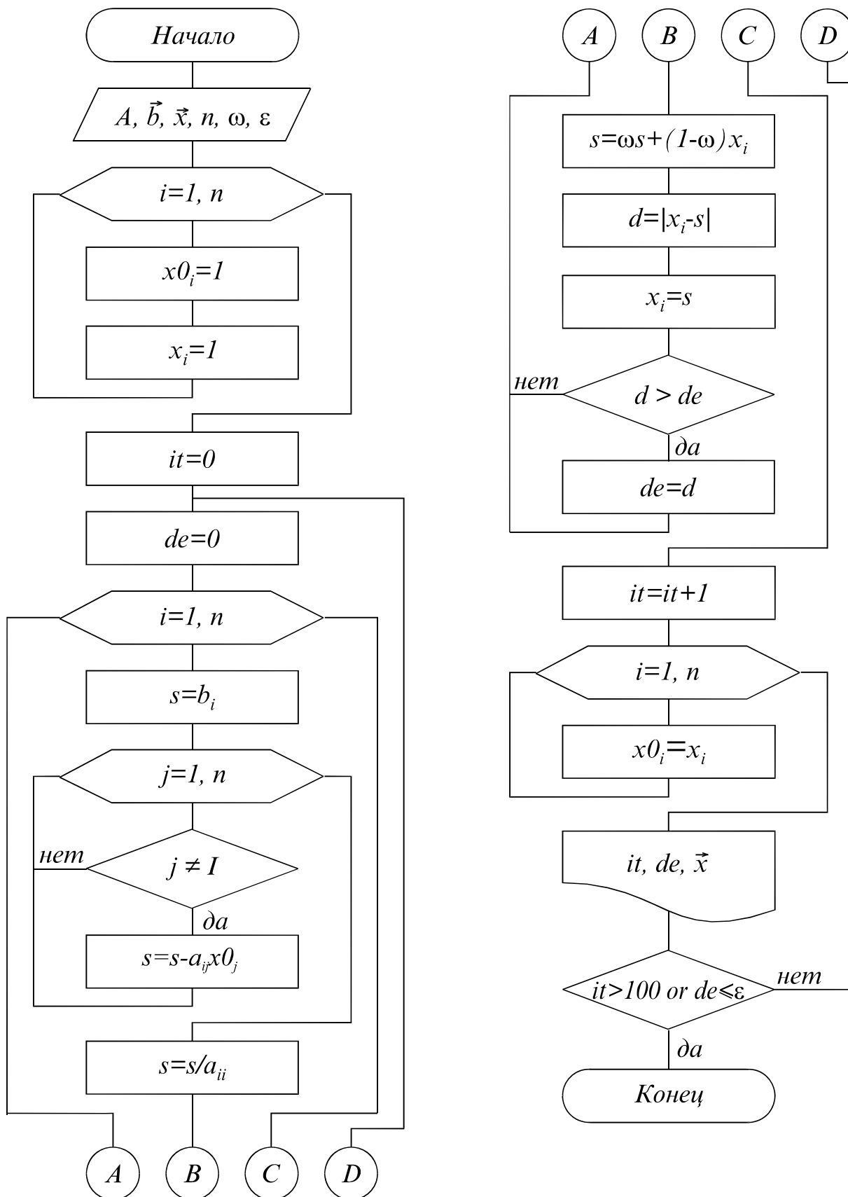
Рис. 15.4 Схема алгоритма метода простой итерации
